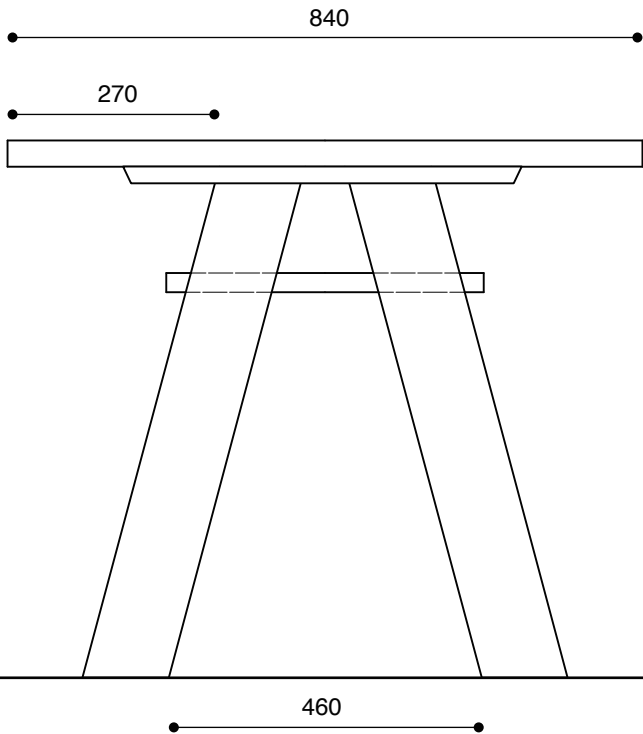
【側面】
